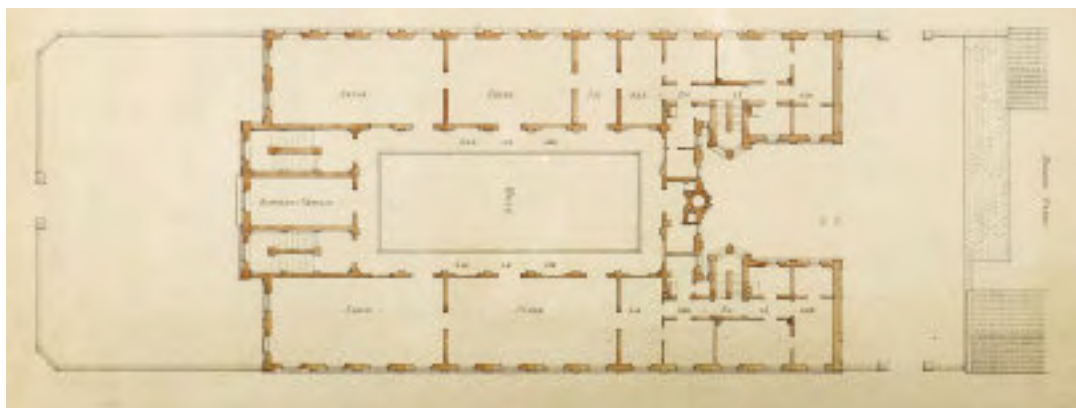
Originale plantegninger. Stueetagen nederst, 1. sal øverst, nord nedad. Omkring aulaen lå skolestuerne, mens lærerboligerne fandtes i bygningens bageste del.
