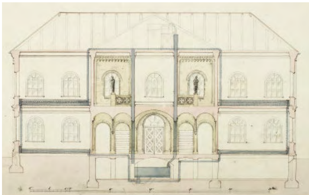
Originaltegning: tværsnit med det for tiden moderne varmeanlæg. Tegningen viser de to oprindelige hovedtrapper på hver sin side af indgangspartiet.
